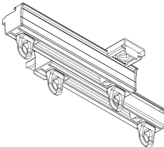
立体图
