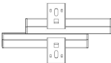
左视图
