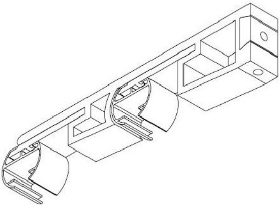
立体图
