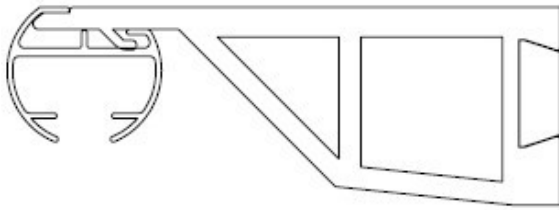
主视图
