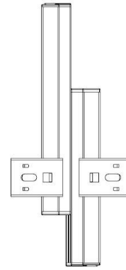
俯视图
